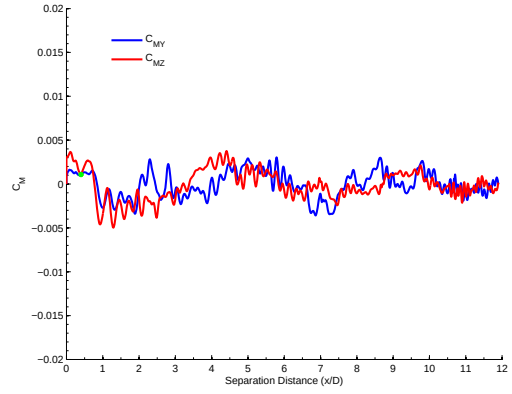
(d) Carrier C_M \gamma = 90^\circ
