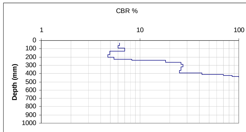
b. 8+50 CL IOP #2 (October 2005).
