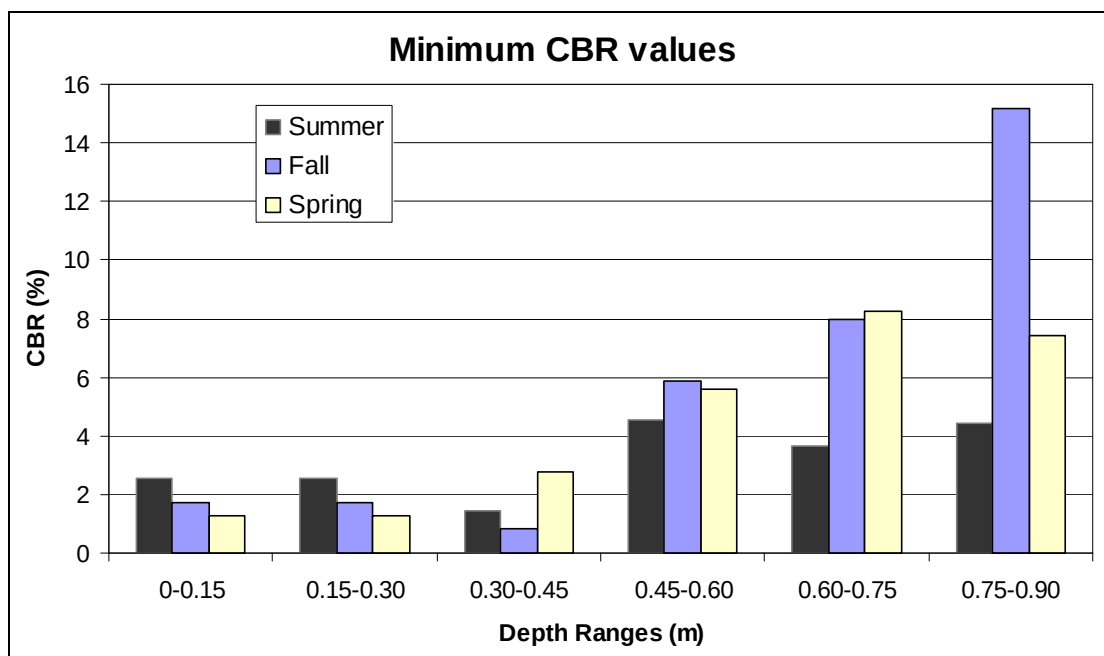
a. Minimum CBR profiles.
