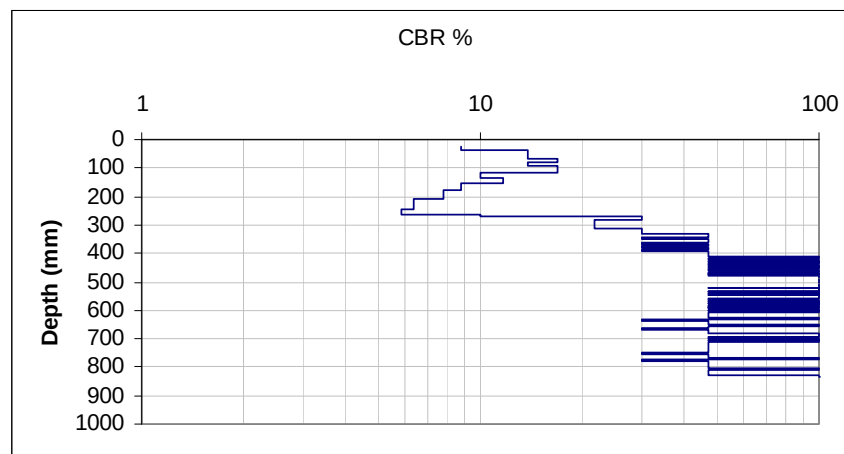
a. 8+50 CL IOP #1 (July 2005).
