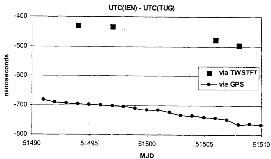
Fig. 10 – UTC(IEN) – UTC(TUG) via TWSTFT and GPS
