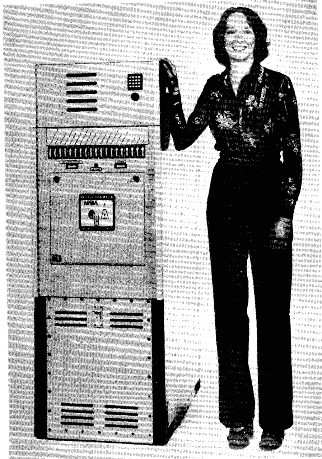
Figure 12. NR Maser
