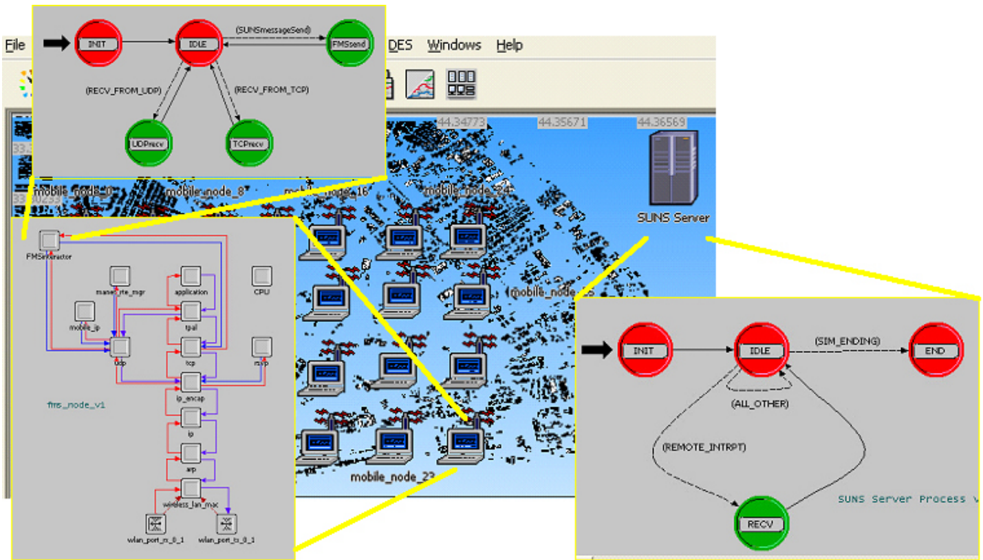
Fig. 2. OPNET models.
