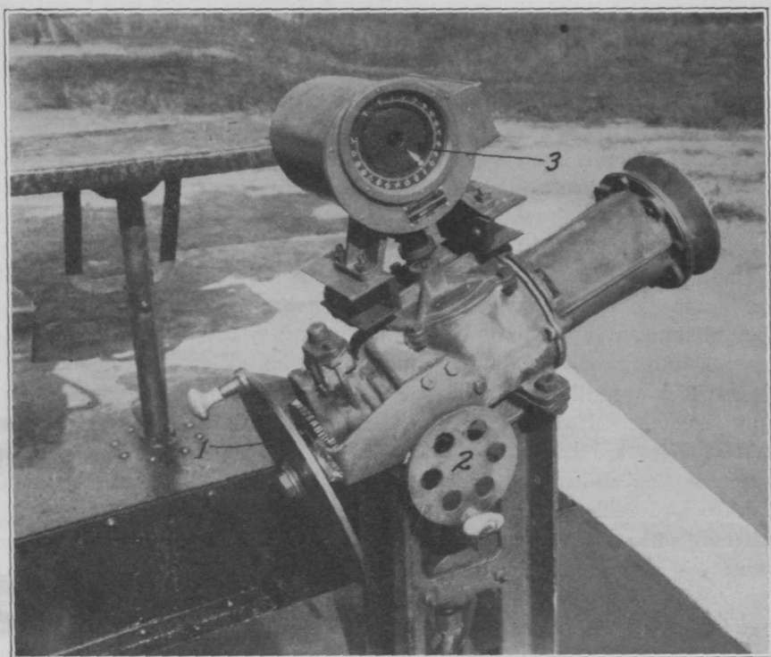
FIG. 6. FUZE SETTER
