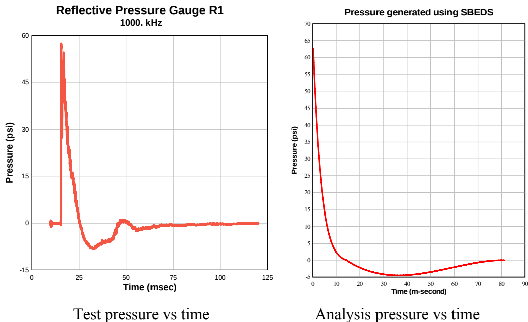
Fig. 9. Blast load for Test 1
