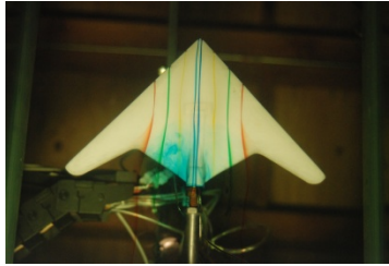
AoA, \alpha=2^\circ
