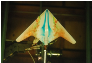
AoA, \alpha=15^\circ
