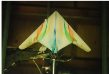
AoA, \alpha=8^\circ
