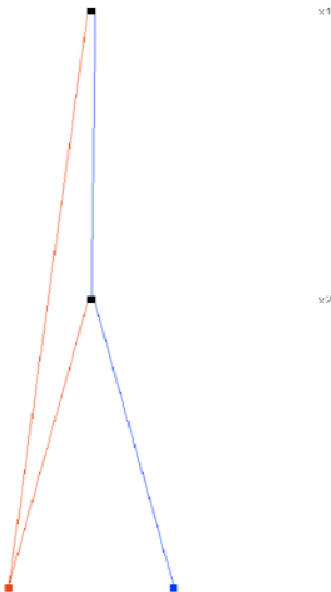
Figure 22. DQF of order 2 ( x_1x_2 ).
