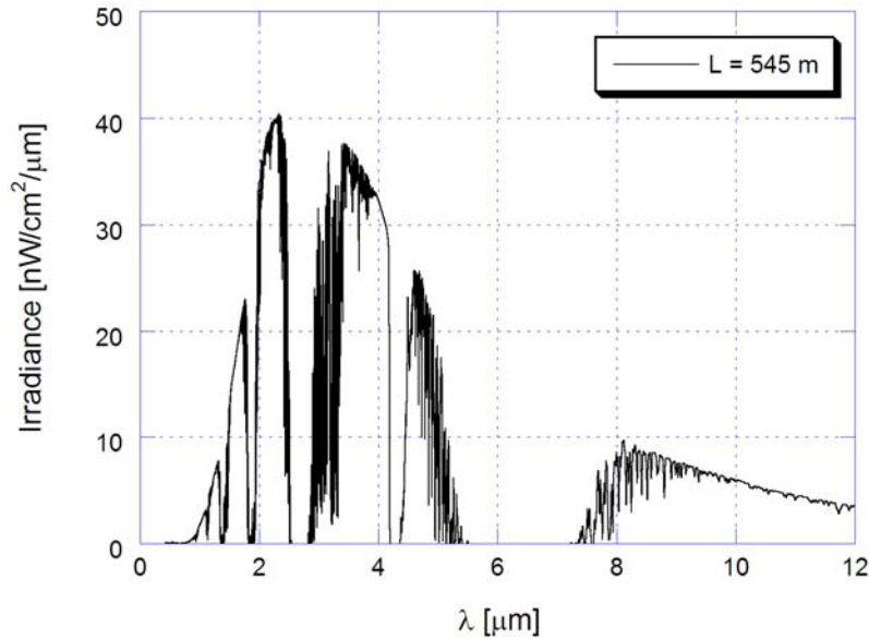
Figure 7. Distribution spectrale d'irradiance à 545 m du radiateur.
