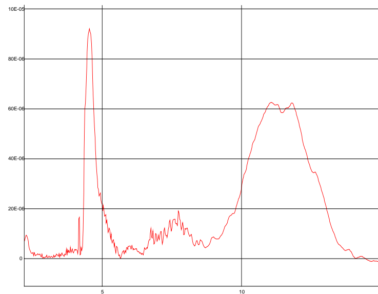
IR SPECTRA
