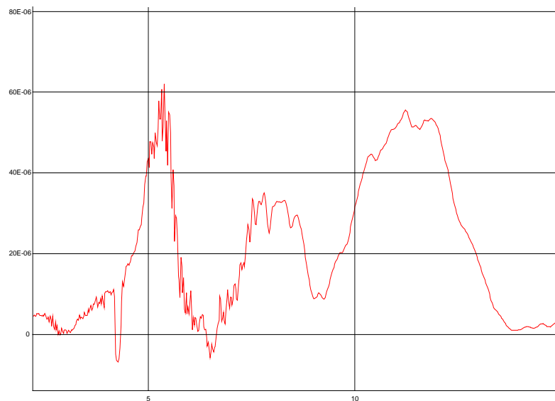
IR SPECTRA
