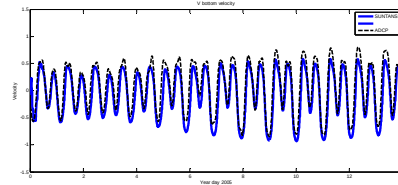
bottom v-velocity
