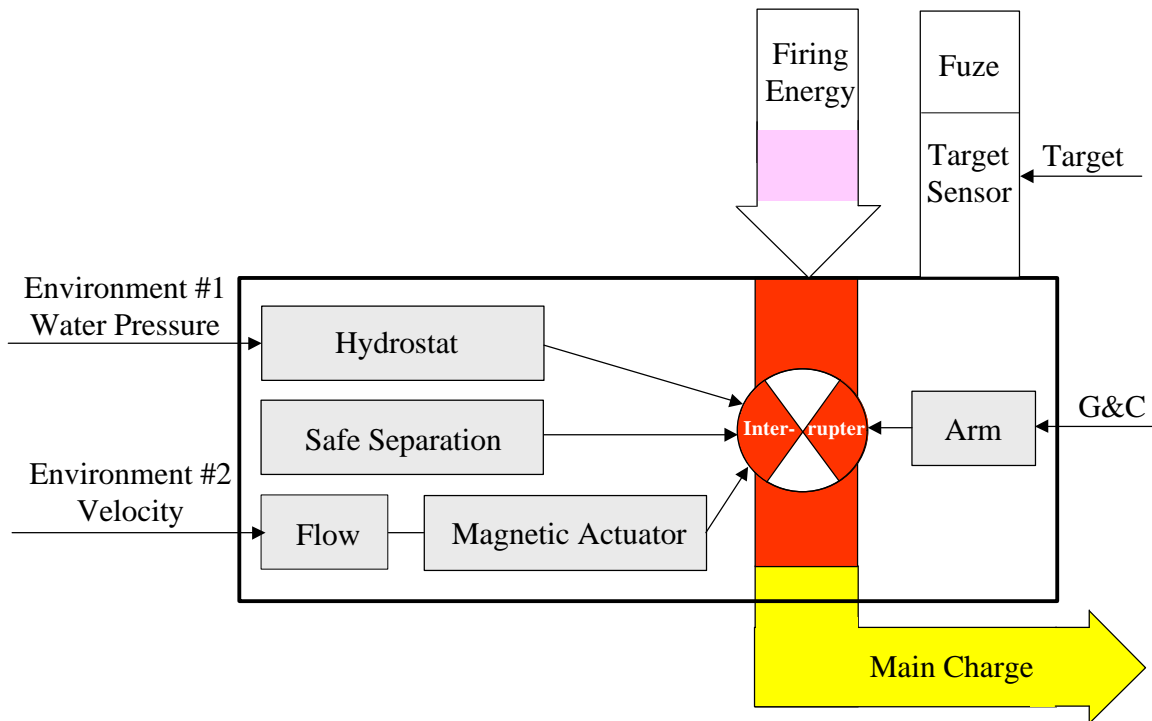
Fig. 3. S&A functional diagram.
