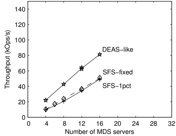
(d) Small constellation NFS throughput
