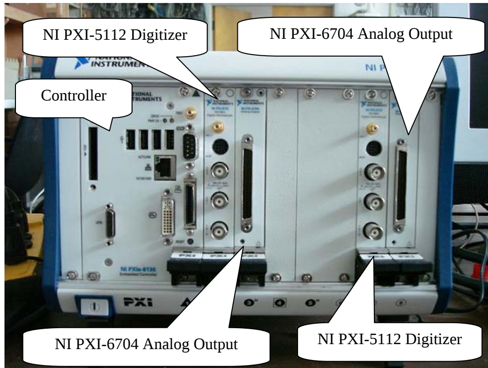
Figure 24. NI PXI-1042 system.
