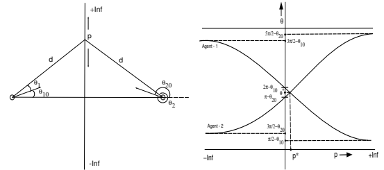
Fig. 2. Voronoi interpretation
