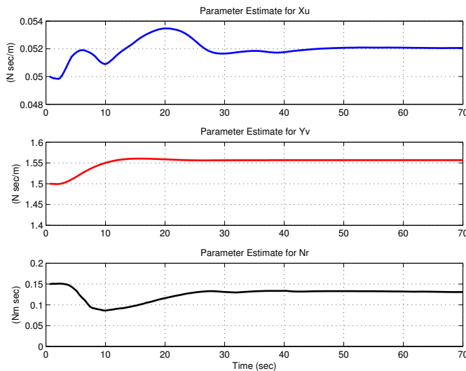
Fig. 6. Parameter Estimates for Drag Effects
