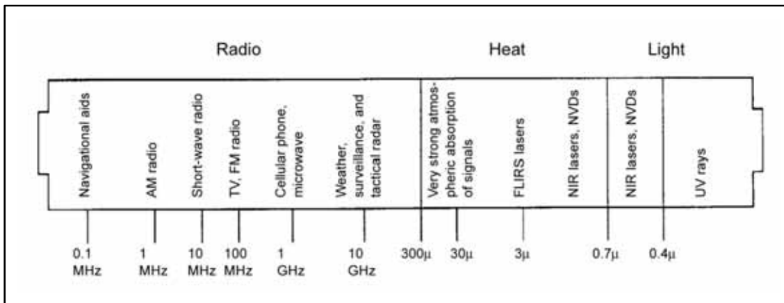
Figure 2-1. EM spectrum
