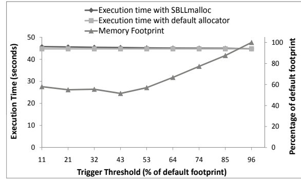
(d) ParaDiS
