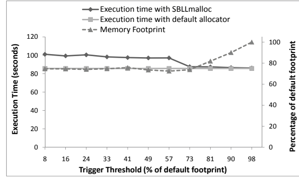
(b) LAMMPS
