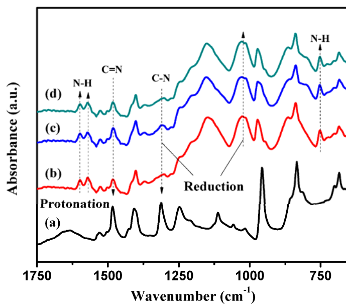
Figure 6 FT-IR spectra of (a) pristine PBZT and PBZT thin film doped with (b) 55 wt% \text{H}_2\text{SO}_4 , (c) 55 wt% \text{H}_2\text{SO}_4 /Fe, and (d) 55 wt% \text{H}_2\text{SO}_4 /Pd.
