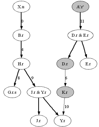
d. \pi_3
