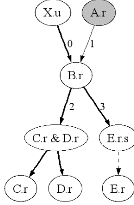
a. \langle \mathcal{P}, \mathcal{R}, X.u \sqsupseteq A.r \rangle
