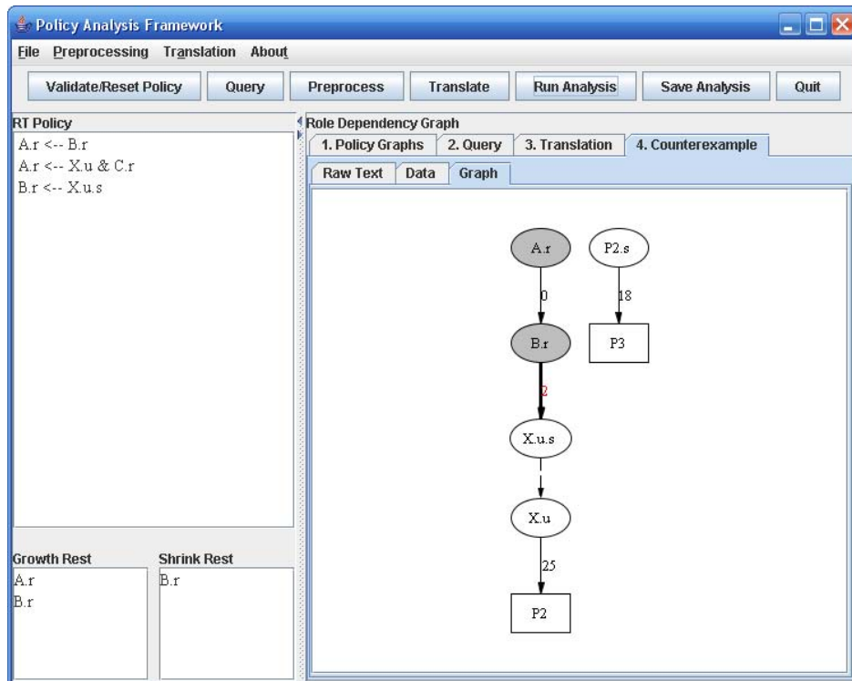
b. Counterexample
