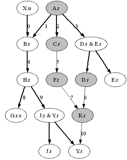
a. \pi
