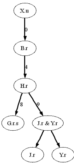
b. \pi_1
