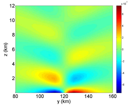
(d) v (m/s) t = 3600 s
