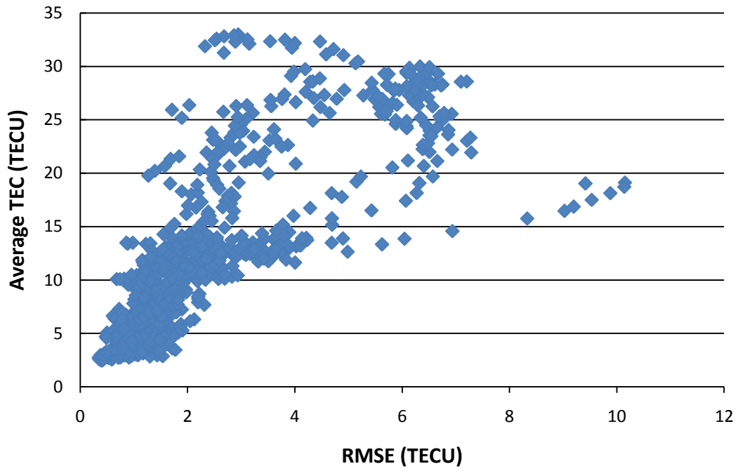
(a) Kp 0-3
