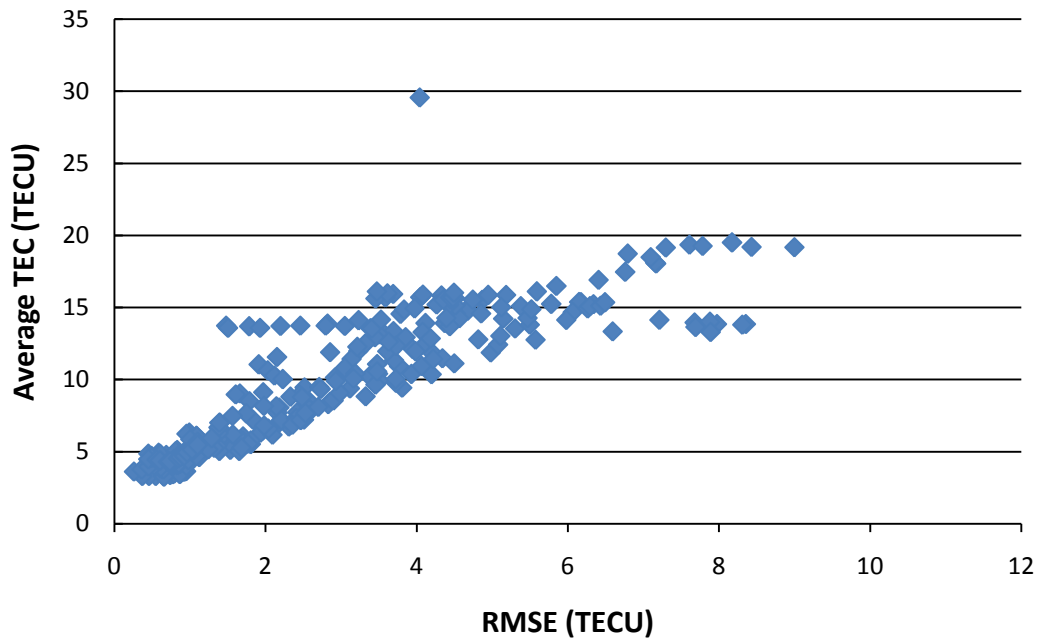
(a) Kp 0-3
