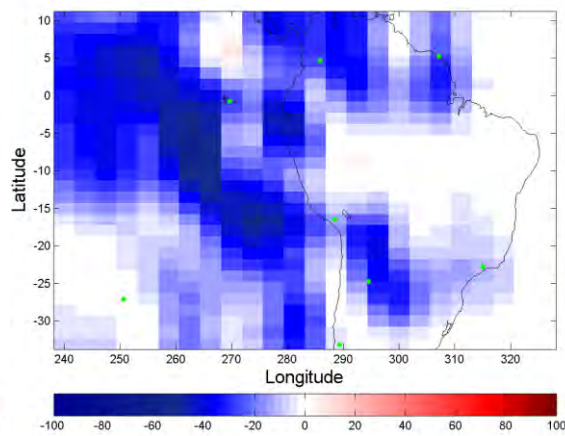
(f) 06UT
