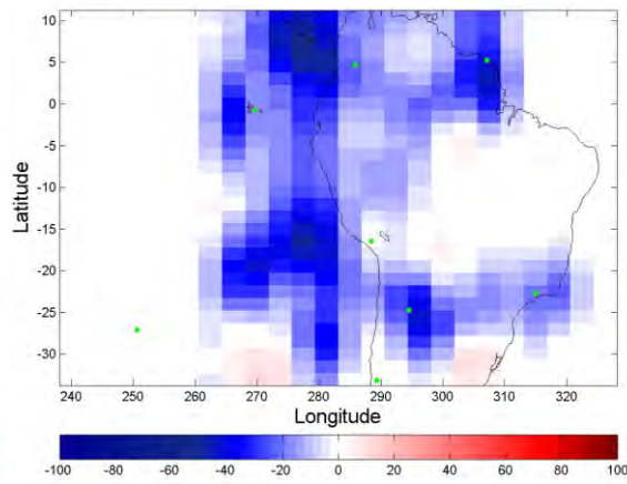
(d) 03UT
