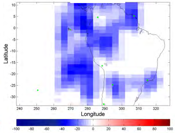
(d) 03UT
