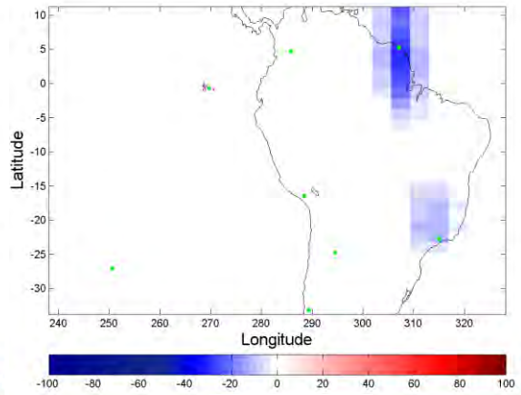
(b) 00UT
