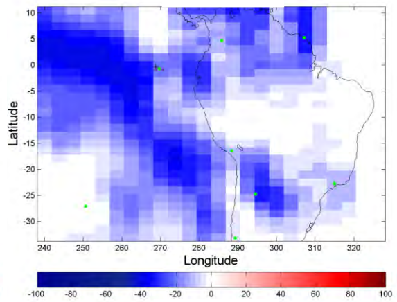
(f) 06UT
