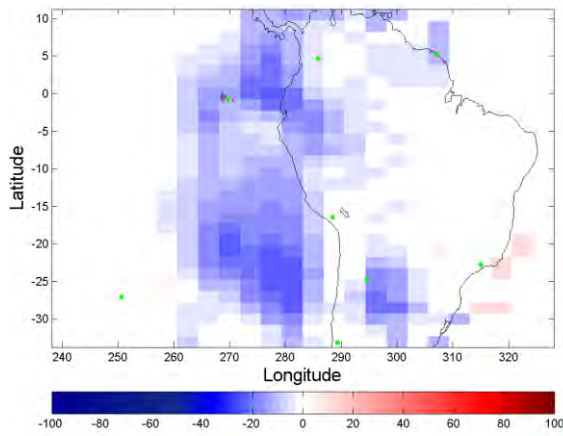
(c) 03UT
