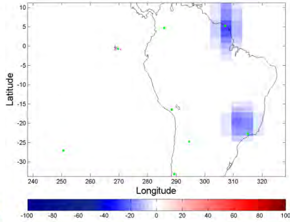
(b) 00UT
