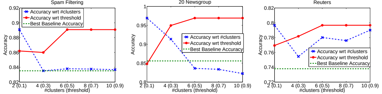
Figure 4.4: Parameter Sensitivity
