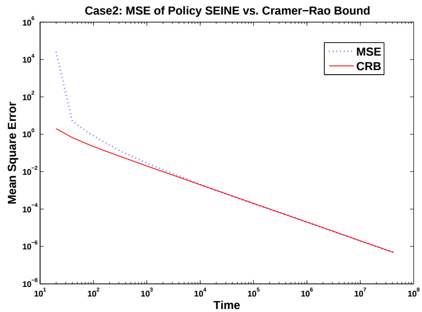
Fig. 9. MSE vs. CRB* : Case 2
