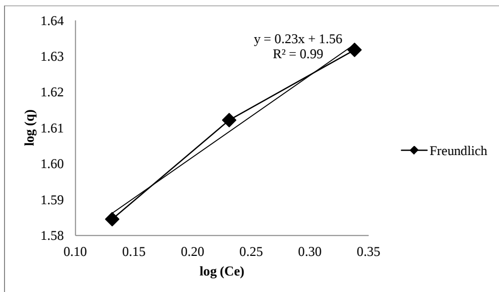
Figure 11. Freundlich Sorption Isotherm: 25 \text{ mg L}^{-1}
