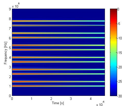
QMFB Layer Q_{23}
