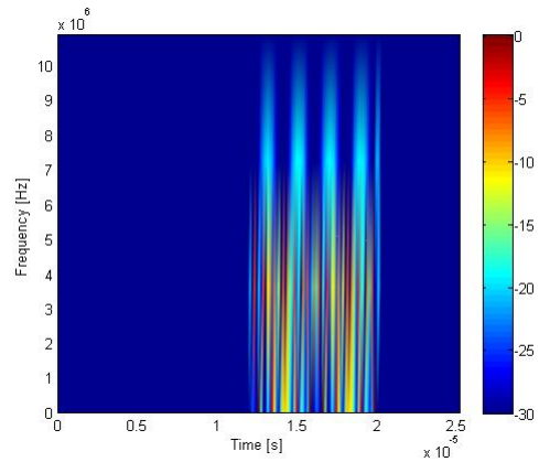
QMFB Layer Q_{15}
