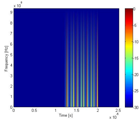
QMFB Layer Q_7
