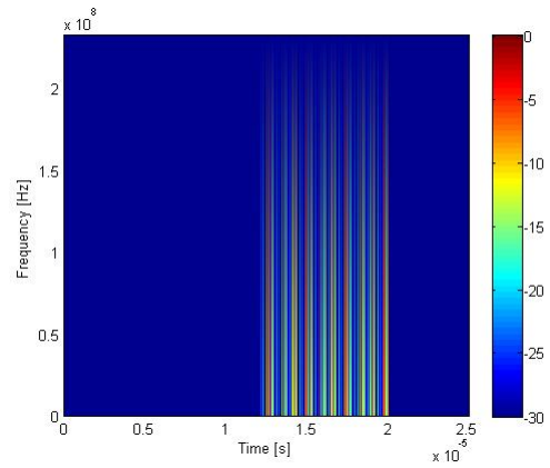
QMFB Layer Q_9
