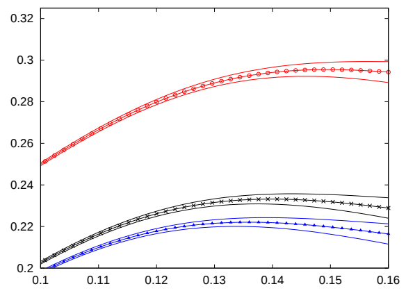
(d) (5000, 0.1) , Zoom near t_f
