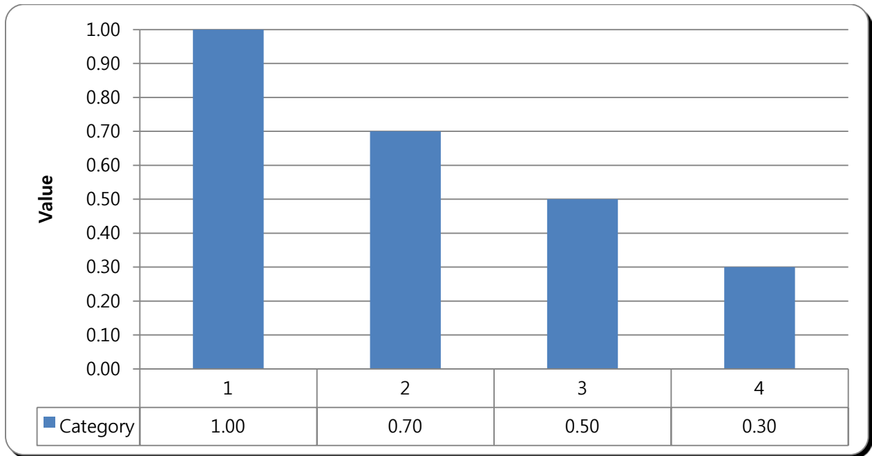
Figure 33 OPR SDVF
