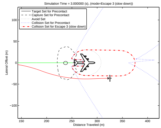
(d) Escape Mode 3 (Slow down), shown at t = 3s
