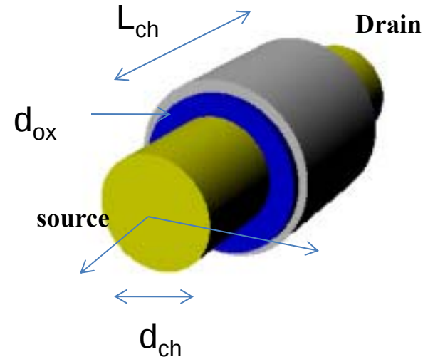
Nanowire MOSFET
