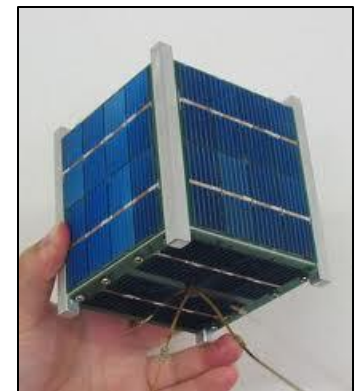
CubeSat 1 kg, 10×10×10 cm
