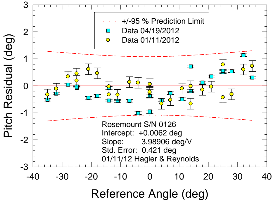
a. Pitch Angle
