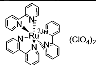
\text{Ru(bpy)}_3(\text{ClO}_4)_2
