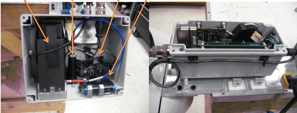
Figure 3b: CULPIS-X V2 sensor package
