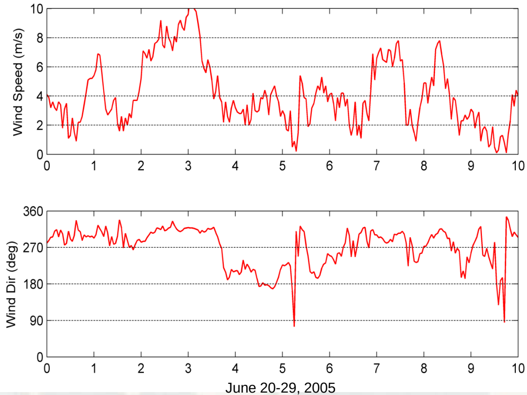
NOAA Buoy 46026
