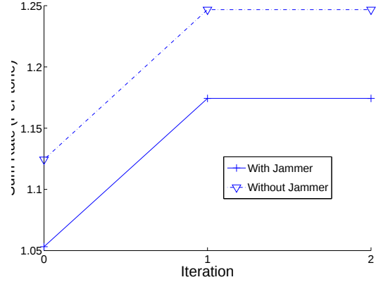
(d) Sum rate with and without a jammer
