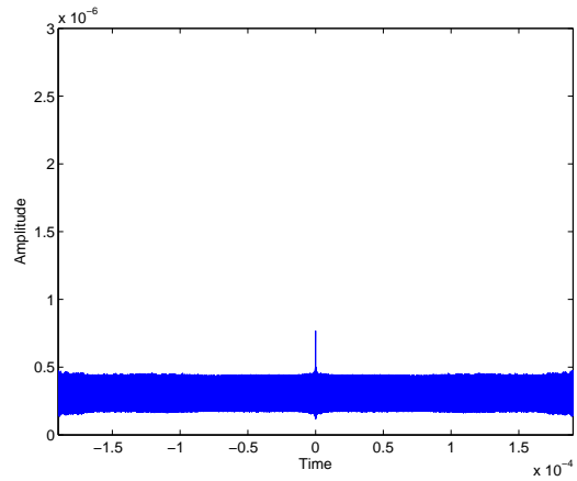
(d) SNIR = -18.03 dB
