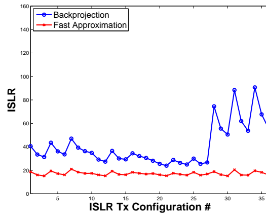
(d) Oversampling by factor of 4
