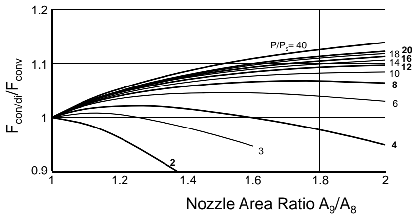
Figure 35: Thrust Ratio Con Di Versus Con Nozzle.
