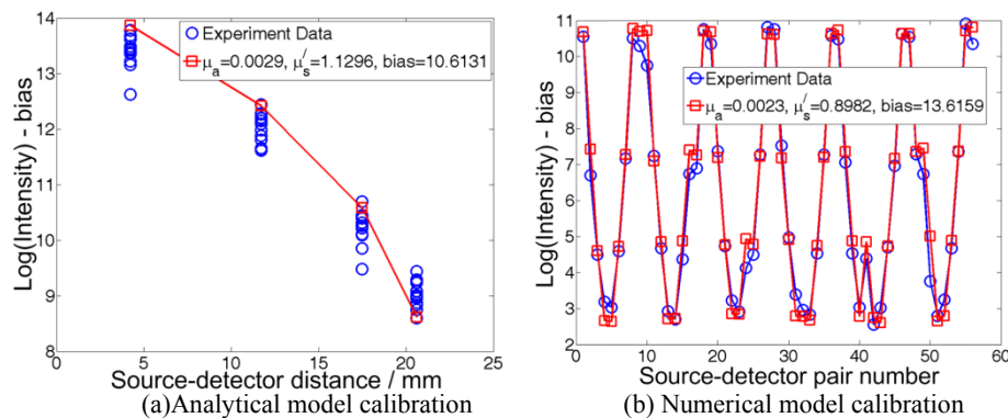
Fig. 5 Data calibration
