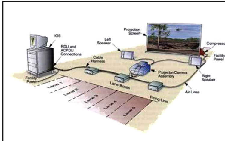
Figure 1. EST 2000 set-up (Anthony, 2006).
