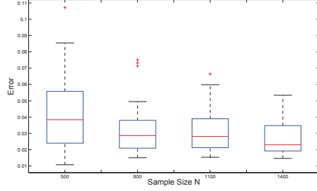
FIG. 4.1. error(x_N^\varepsilon) when \varepsilon = 0.2 .
