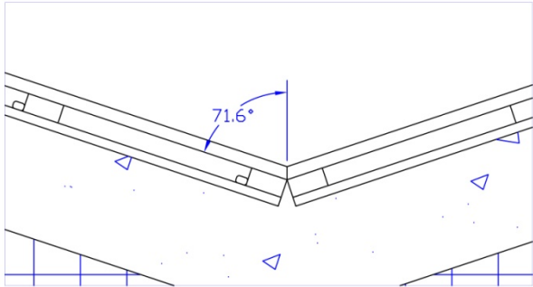
DETAIL 3 (SCALE: 1:4)
