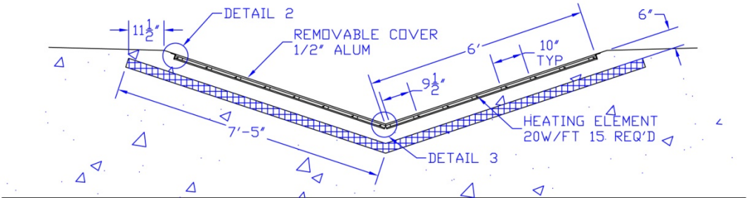
DETAIL 1 (SCALE: 1:25)
