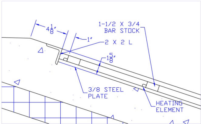
DETAIL 2 (SCALE: 1:4)
