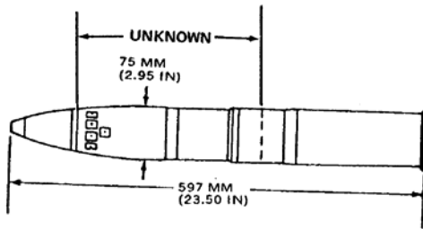
Projectile, 75 mm, HEAT. M66
