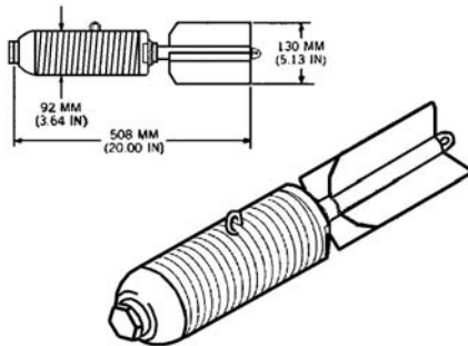
Bomb, 20-lb, Fragmentation, AN-M41; AN-M41A1
