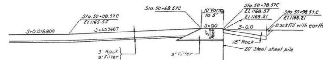
SECTION D-D
