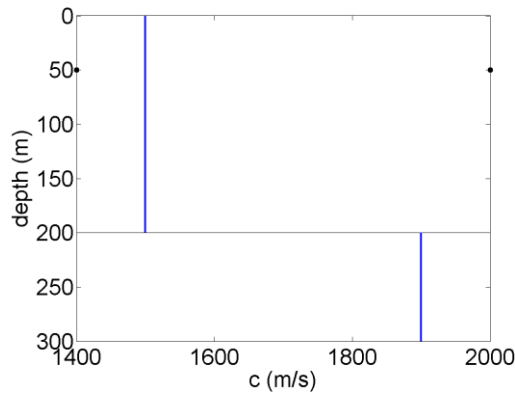
Fig. 1. Pekeris waveguide
