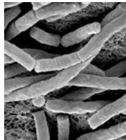
Pseudonocardia Dioxanivorans (CB1190)
