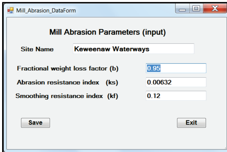
Figure 12. Mill abrasion input data.
